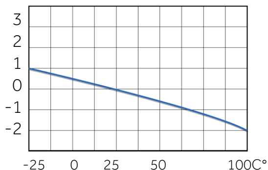
Delta C/C %
